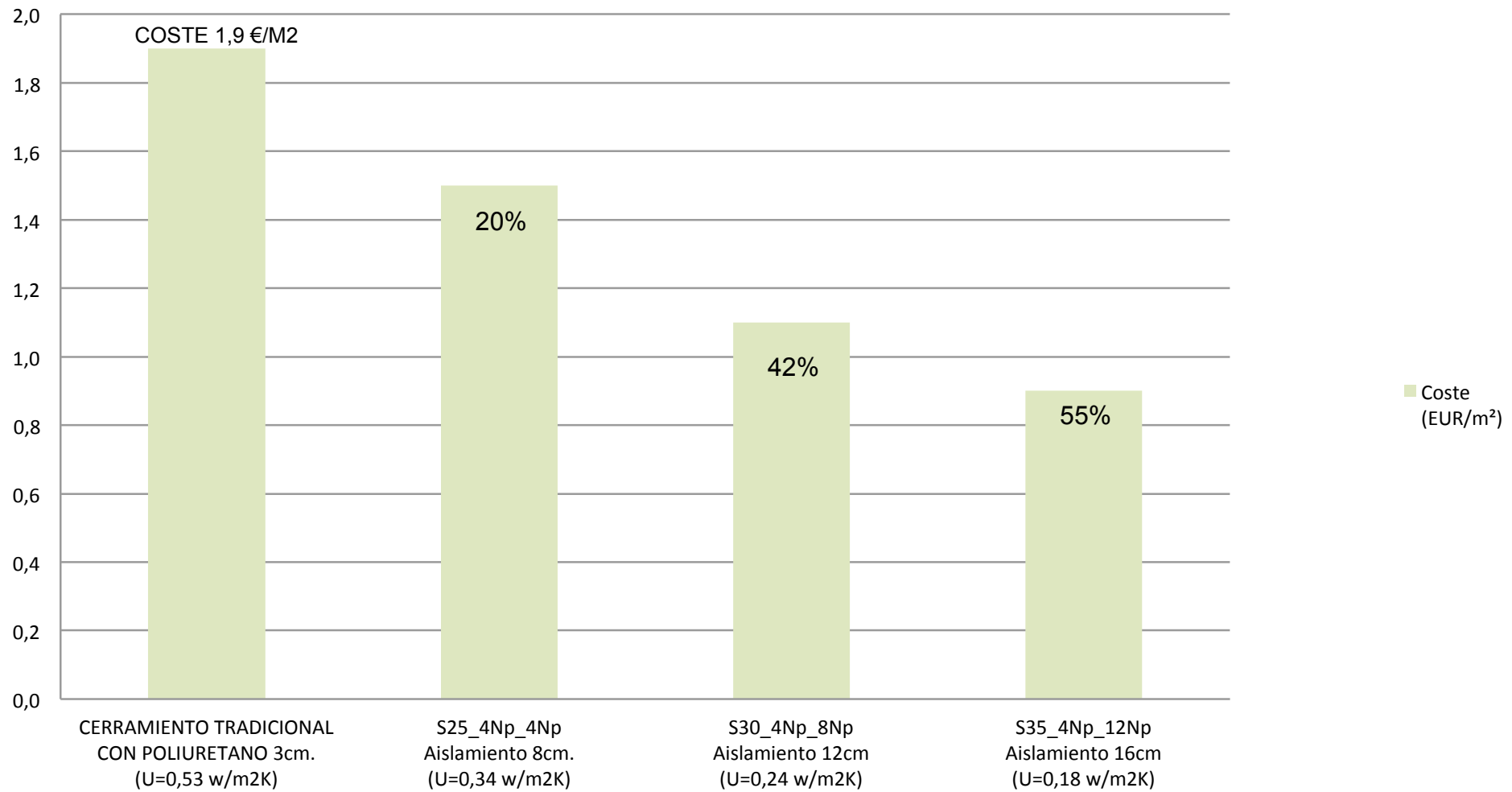
Coste Energético según tipo Muro Cerramiento (EUR/m 2 )
